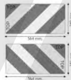
Schema per l'installazione Installation scheme
