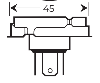
P45t IEC 7004-95 DIN 49737
